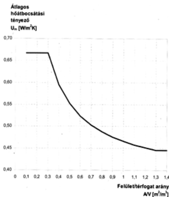
2. ábra: Az átlagos hőátbocsátási tényező követelményértékei
