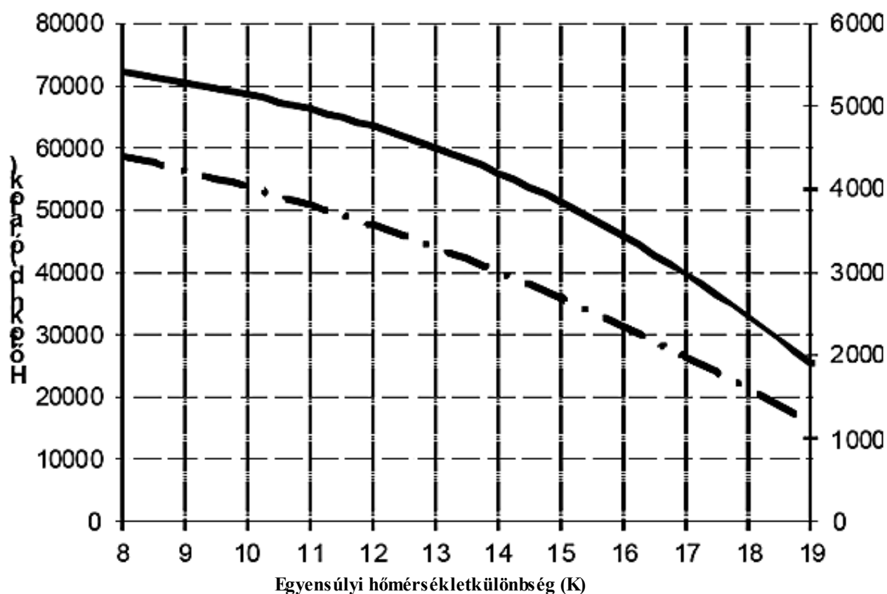
1. ábra: Hőfokhid és fűtési idény hossza 20 °C belső hőmérséklet esetén az egyensúlyi hőmérsékletkülönbség függvényében
